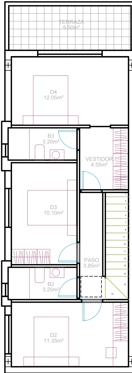
PLANTA PRIMERA
