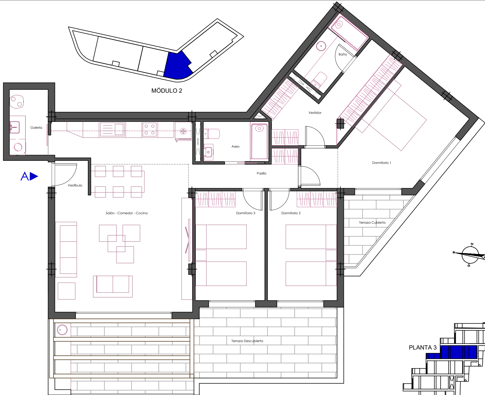
MÓDULO 2. PLANTA 3. Vivienda A.
